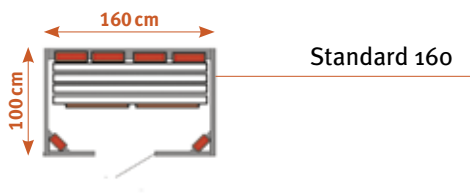
Standard 160 mit Klappbank
